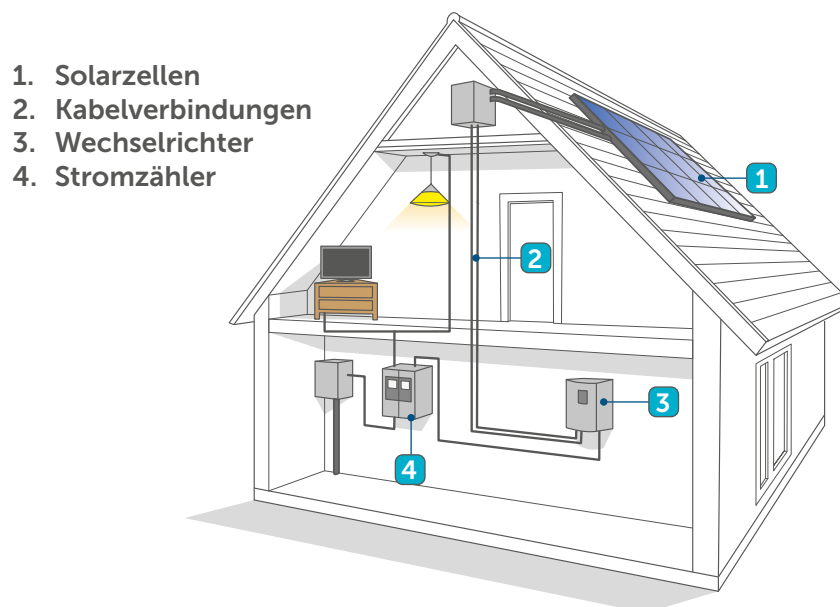
Abbildung 7: Haus mit PV-Anlage und Zähler
